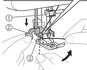
① Porte-aiguille ② Levier de l'enfile-aiguille ③ Guide
