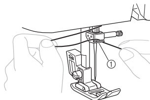
① Guide-fil de la barre à aiguille
