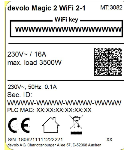
Fig. 4 : Plaque signalétique
